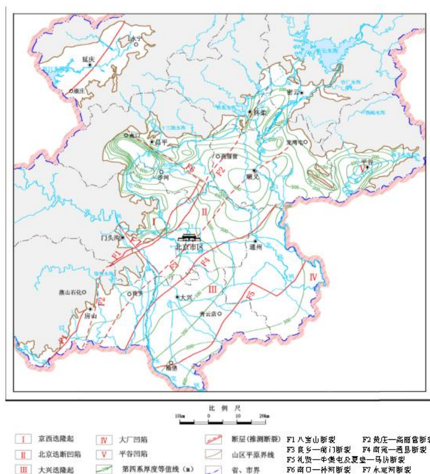
图 1.2-3 北京平原区断裂构造略图
